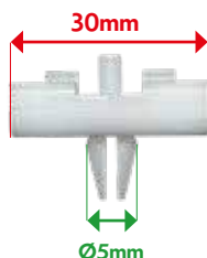
VB12036 GLAZING CLIP R50, R52 et R53
