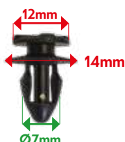
VB82327 TRIM CLIP Laguna, Laguna Nevada, Safrane
