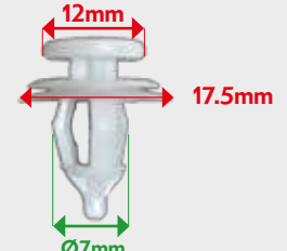
VB72205 TRIM CLIP Berlingo, Picasso et Saxo
