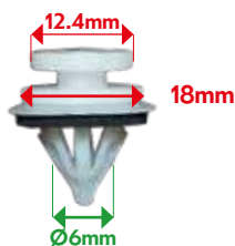
VB93305 TRIM CLIP C4 Picasso
