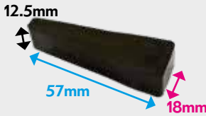
VB4000501 RUBBER WEDGE Coccinelle (11-), Scirocco III (08-)
