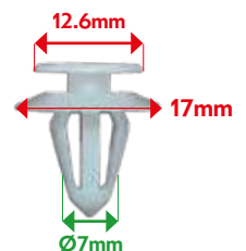
VB56305 TRIM CLIP
