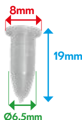
VB89427 TRIM CLIP BUSH Ulysse et Scudo
