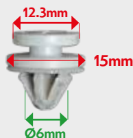
VB18255 TRIM CLIP Clio I, Megane, Trafic
