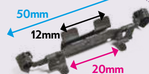
VB4000110 METAL TRIM CLIP Trafic - Clio 3
