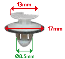
VB20305 TRIM CLIP
