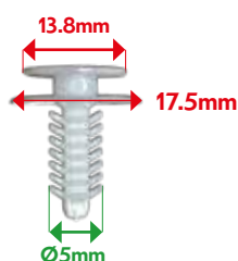
VB59405 TRIM CLIP Brava, Bravo, Doblo, Marea, Punto (99-03), Palio, Siena, Stilo, Strada, Tempra, Tipo, Panda <03, Punto 03...
