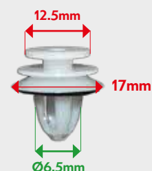
VB3101007 WINDSHIELD CLIP A PILLAR R56 (07-), R57 (09-), cabrio et Clubman R55 (08-), R50, R53 et cabrio R52 (01-06)
